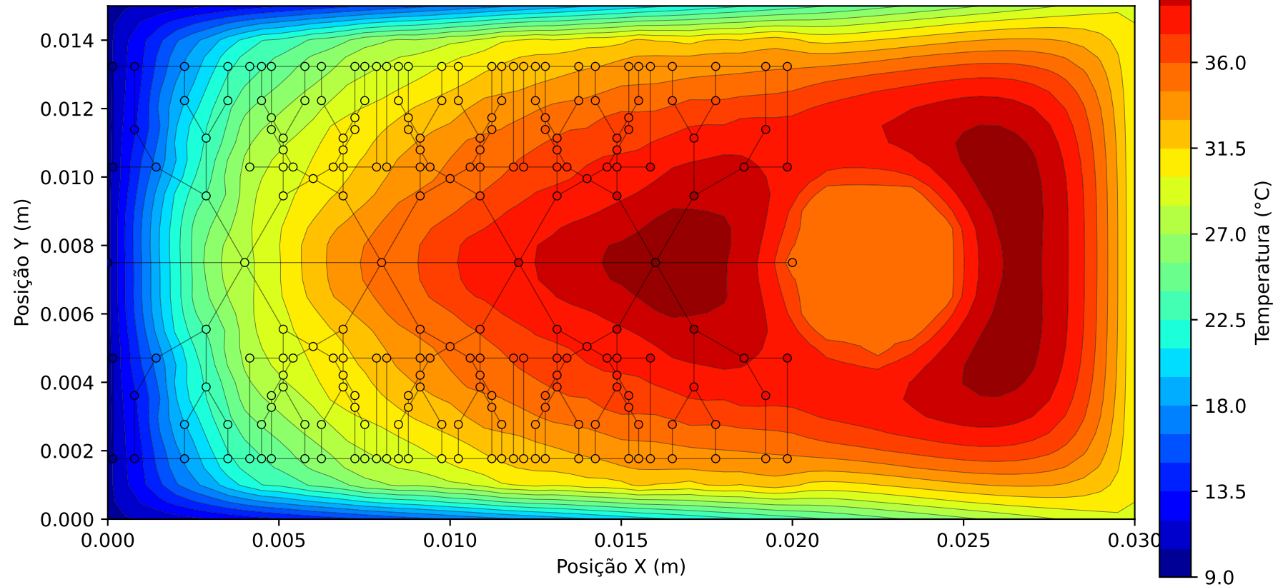
Campo Térmico 2D - Malha 61x31 | d_{max} = 0.0005 m
