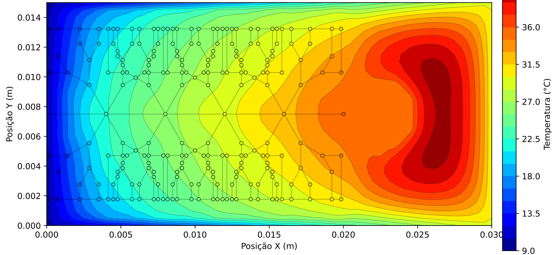
Campo Térmico 2D - Malha 61x31 | d_{max} = 0.001 m
