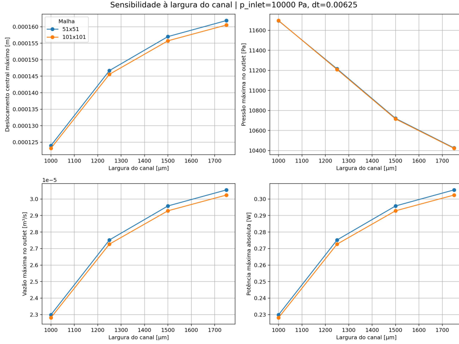
Figura 39: Sensibilidade à largura do canal, H_k \in \{1000, 1250, 1500, 1750\} \mu\text{m} .
