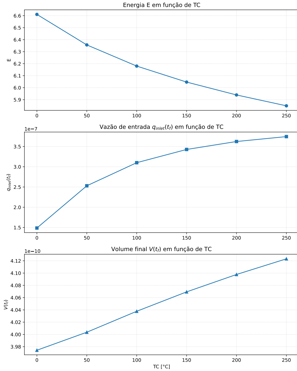
Figura 52: Evolução dos indicadores de Energia, Vazão de entrada final e Volume final em função da temperatura da inclusão circular ( T_C ).
