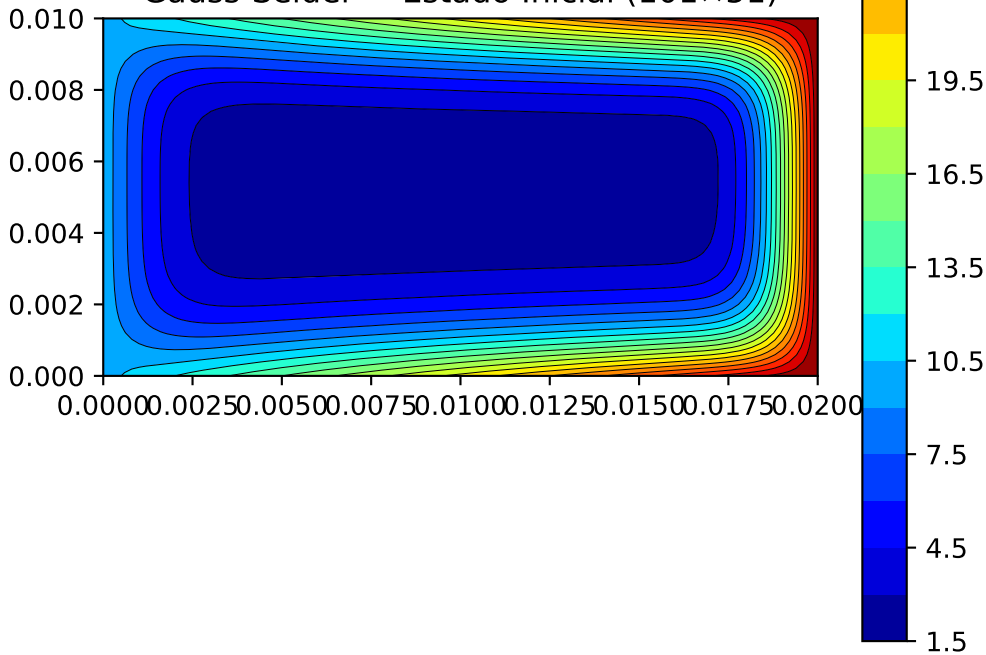
Gauss-Seidel — Estado Inicial (101×51)
