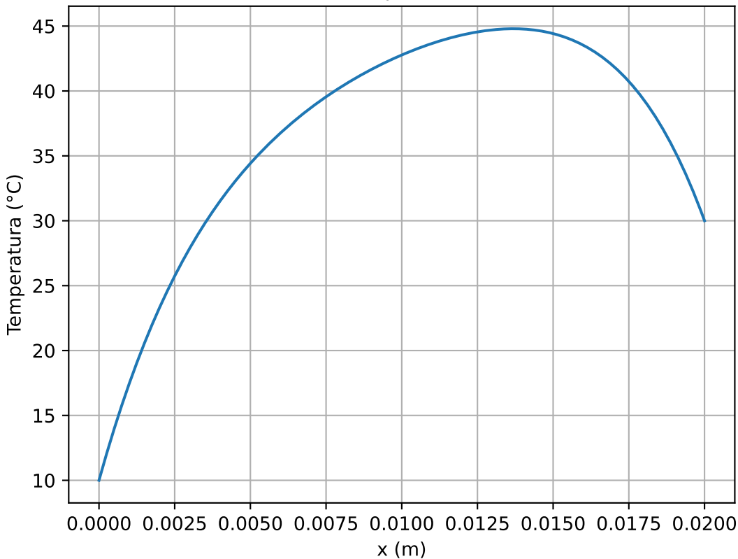
Eixo Central (161 X 81) | Temp. Máxima: 44.794 °C
