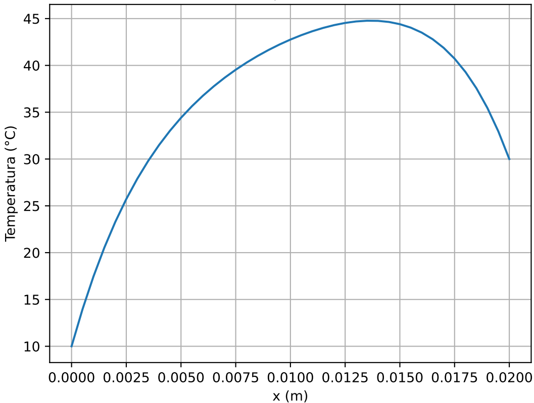
Eixo Central (41 X 21) | Temp. Máxima: 44.773 °C
