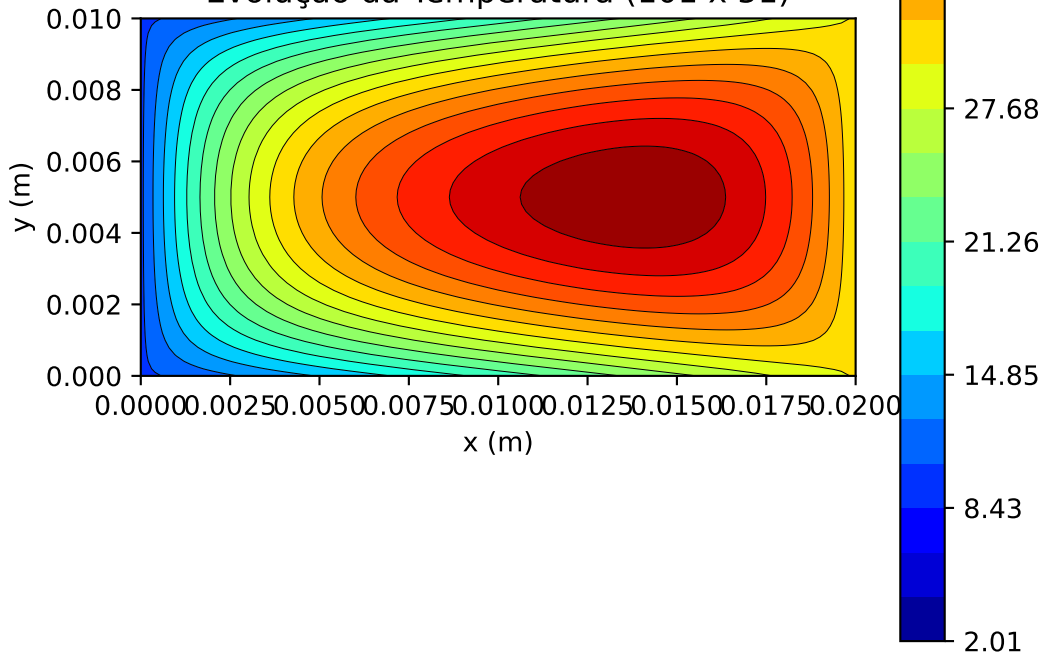
Evolução da Temperatura (101 x 51)
