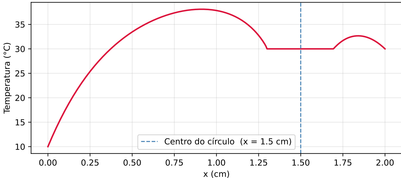
Perfil de temperatura - eixo central (321×161)
