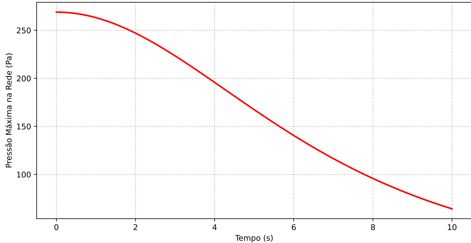
Efeito do Aquecimento na Pressão Máxima (Item 6 - Otimizado)
