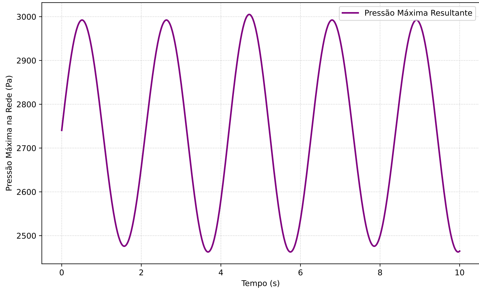
Pressão Máxima na Rede (Itens 4 e 5 - Superposição)
