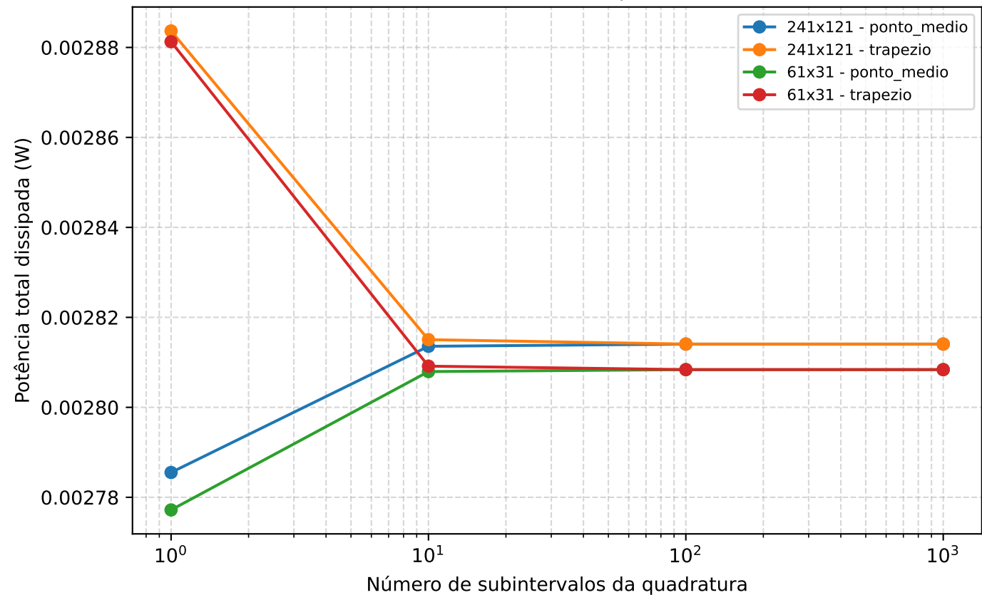
Potência total em função da quadratura térmica
