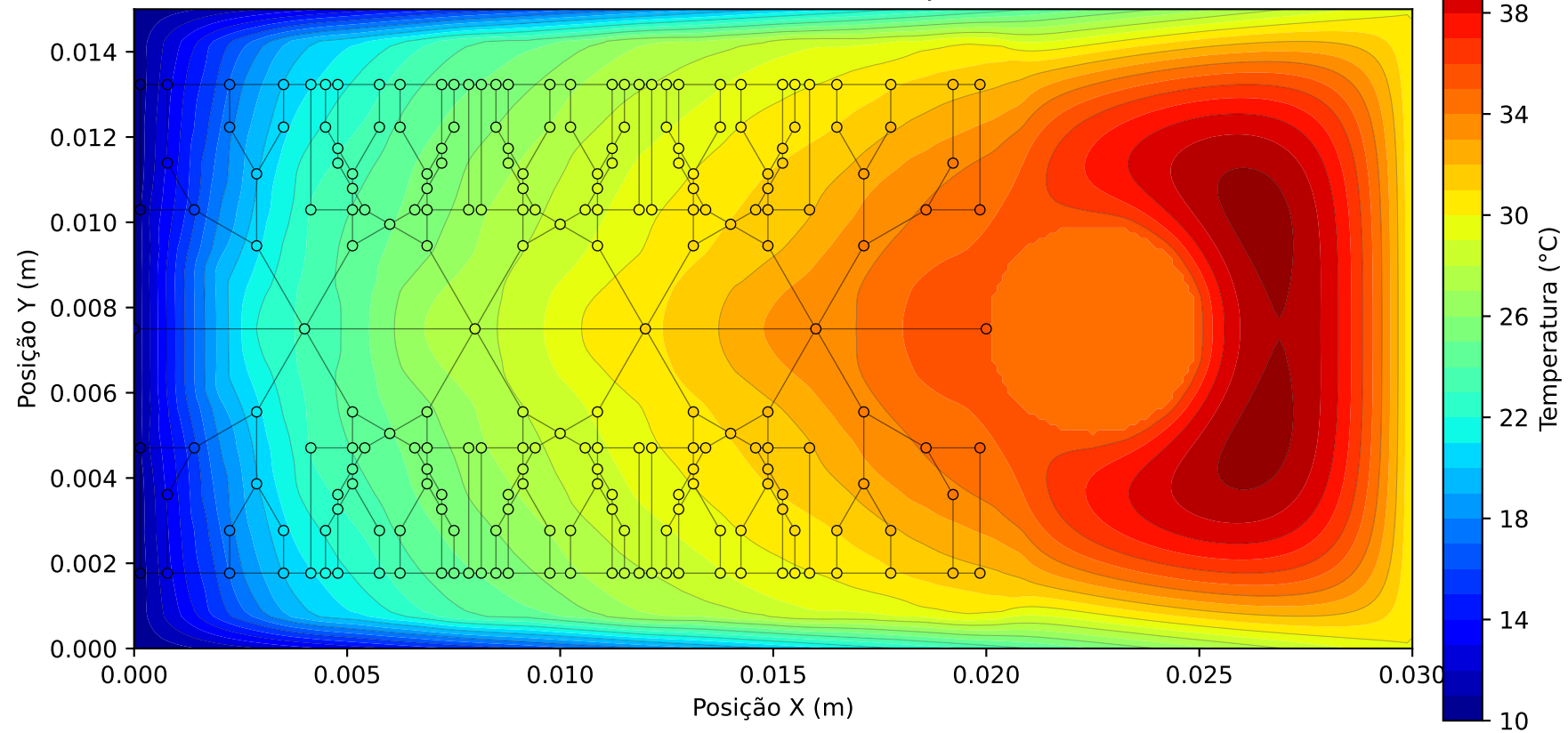
Campo Térmico 2D - Malha 241x121 | d_{max} = 0.001 m
