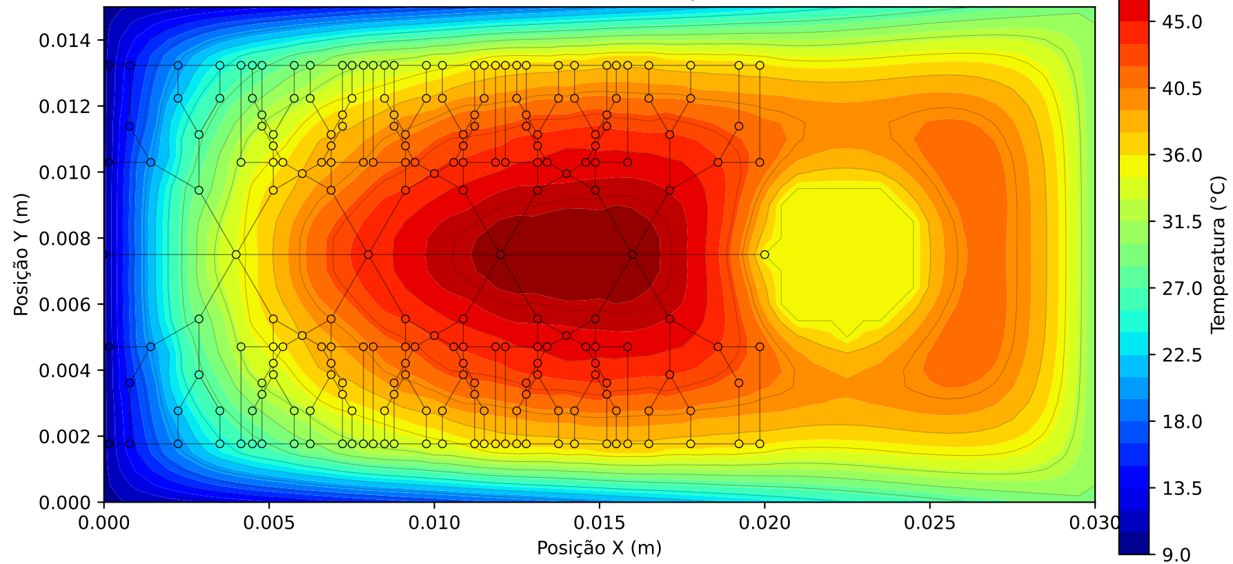
Campo Térmico 2D - Malha 61x31 | d_{max} = 0.00025 m
