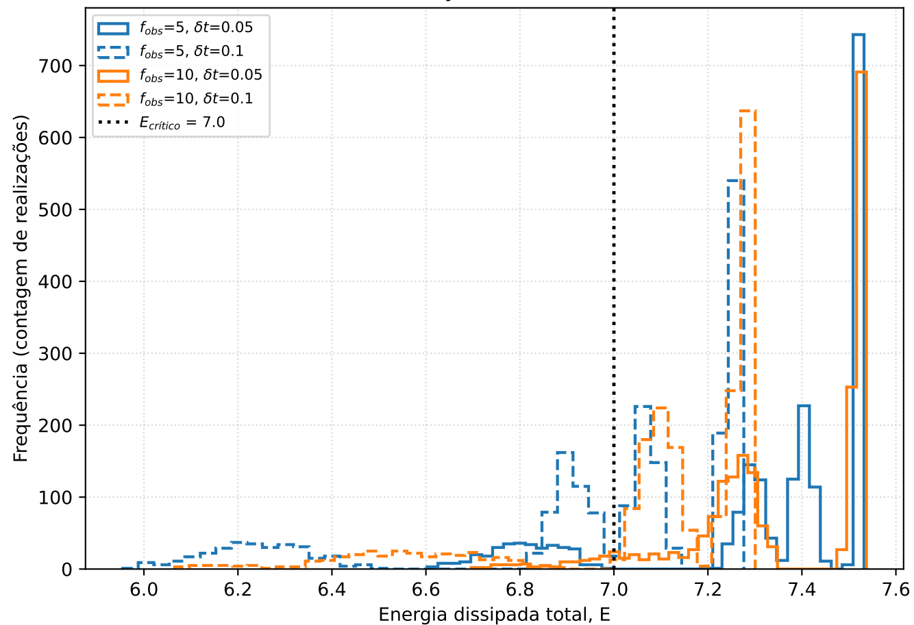
Distribuição amostral de E
