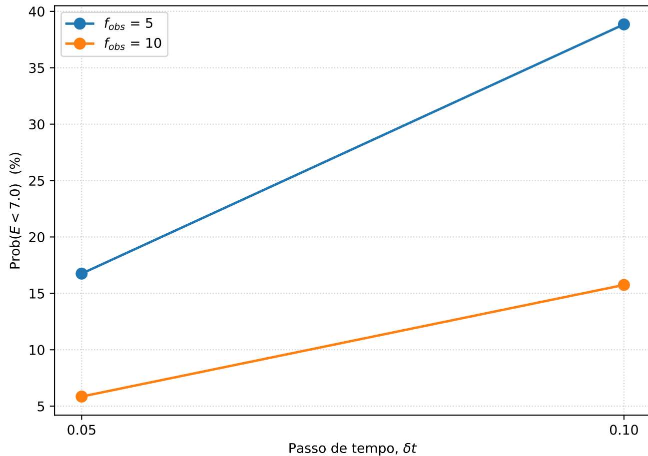
Análise Dinâmica do GD Completo ( p_O=0.6 , N=2000 por ponto)
