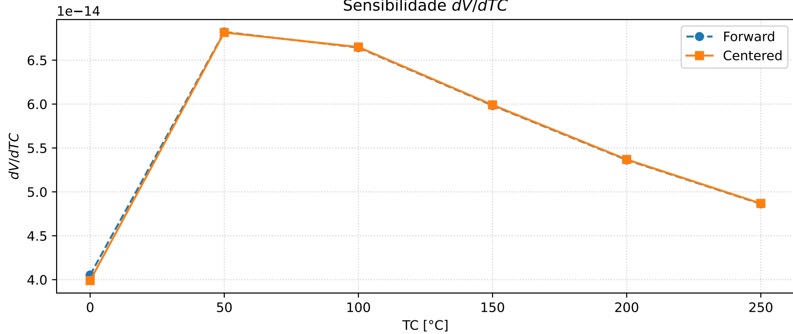
Sensibilidade dV/dTC
