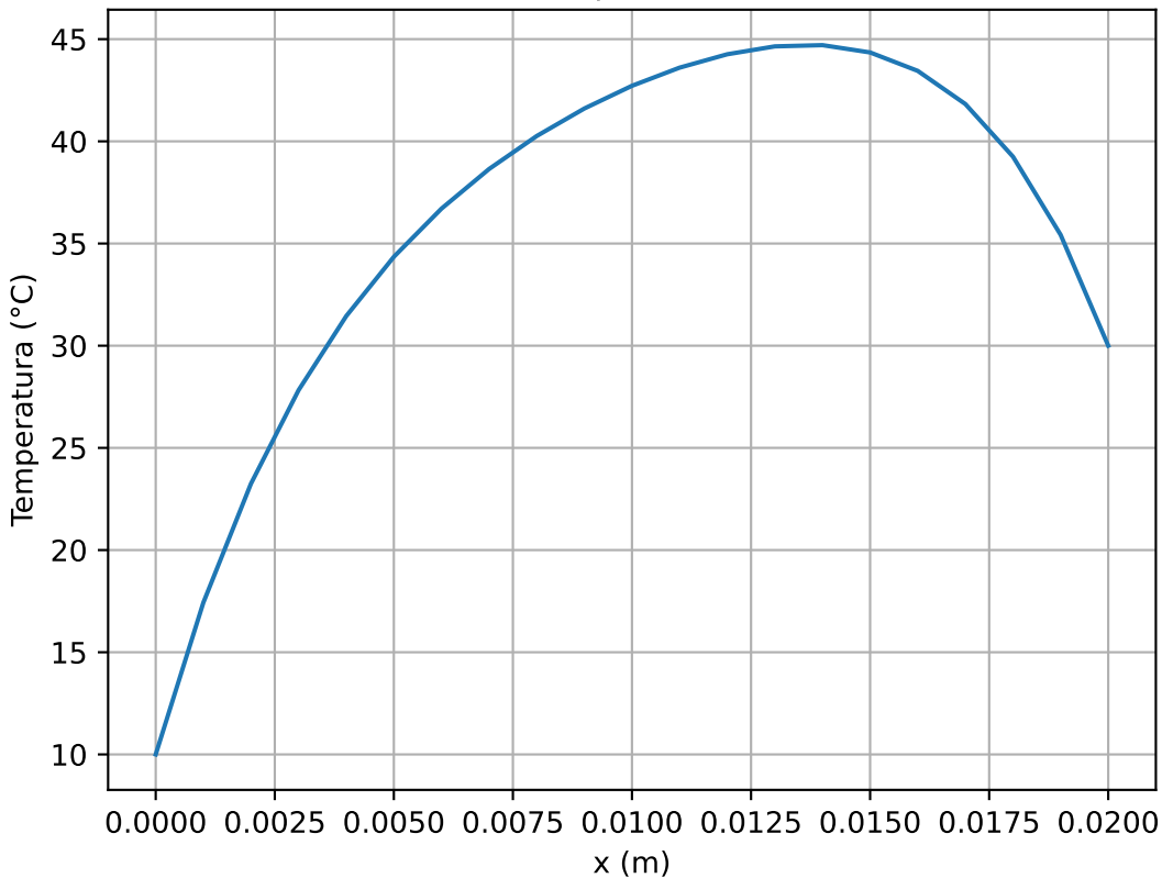
Eixo Central (21 X 11) | Temp. Máxima: 44.707 °C
