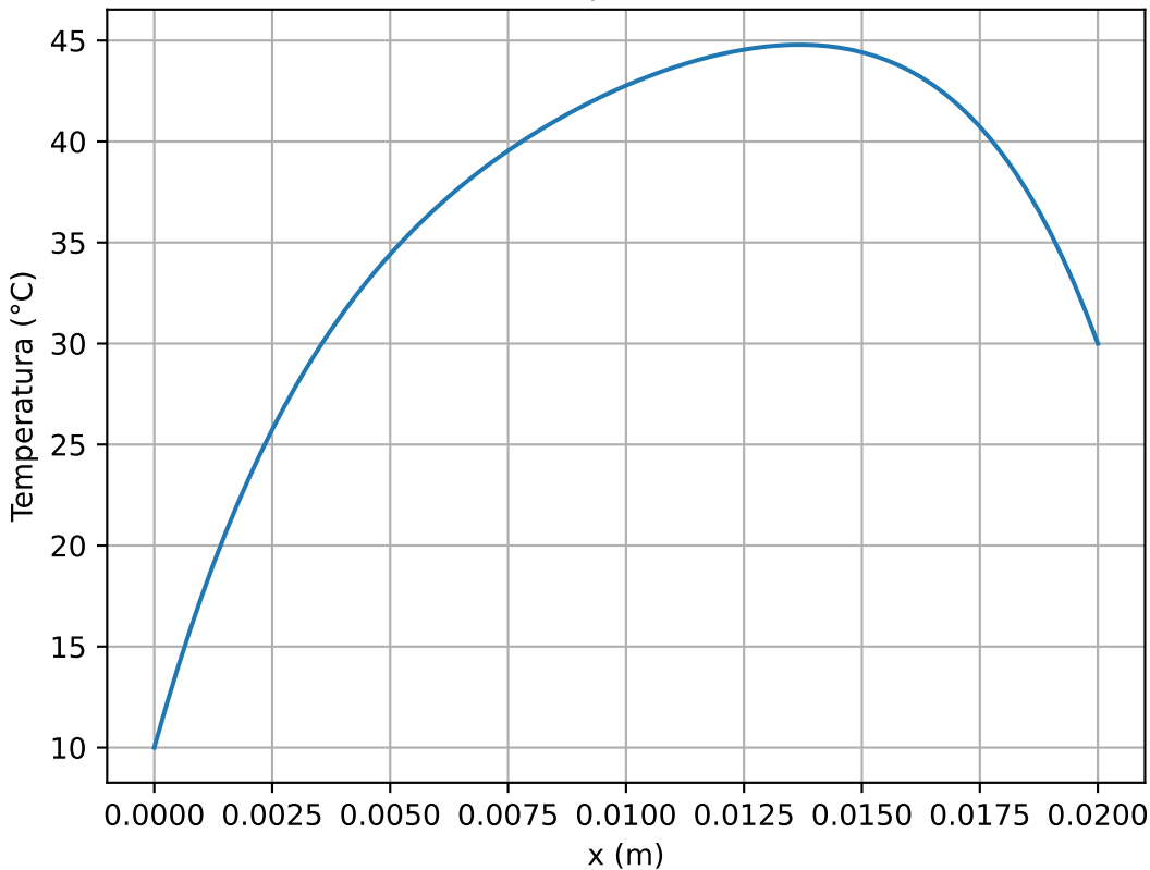
Eixo Central (81 X 41) | Temp. Máxima: 44.791 °C
