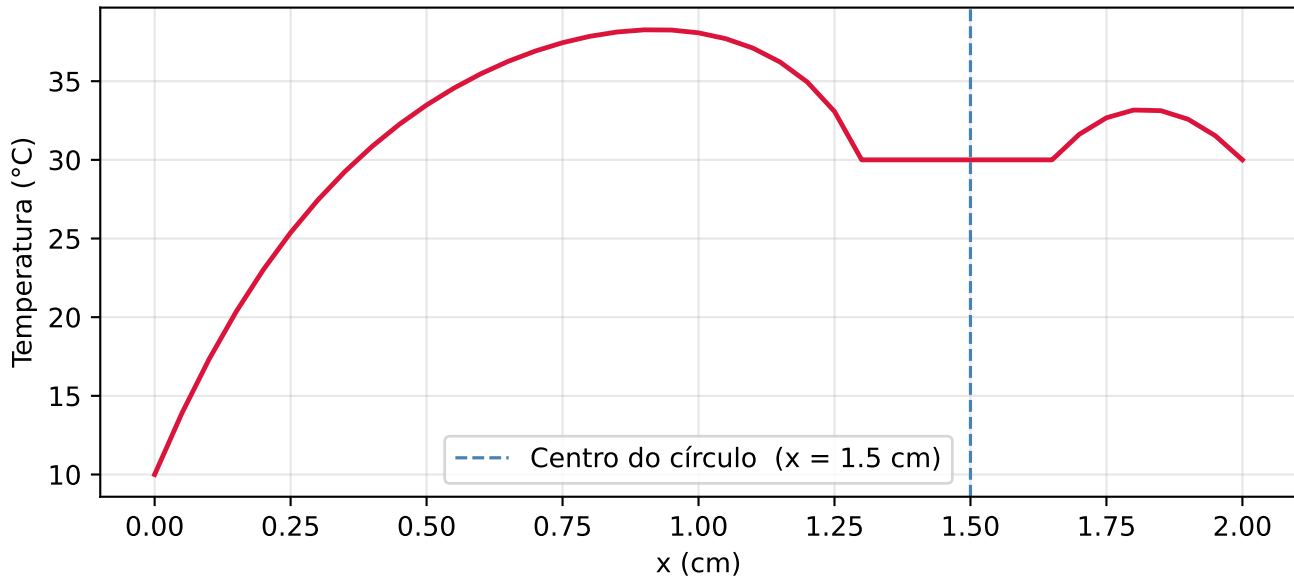
Perfil de temperatura - eixo central (41×21)
