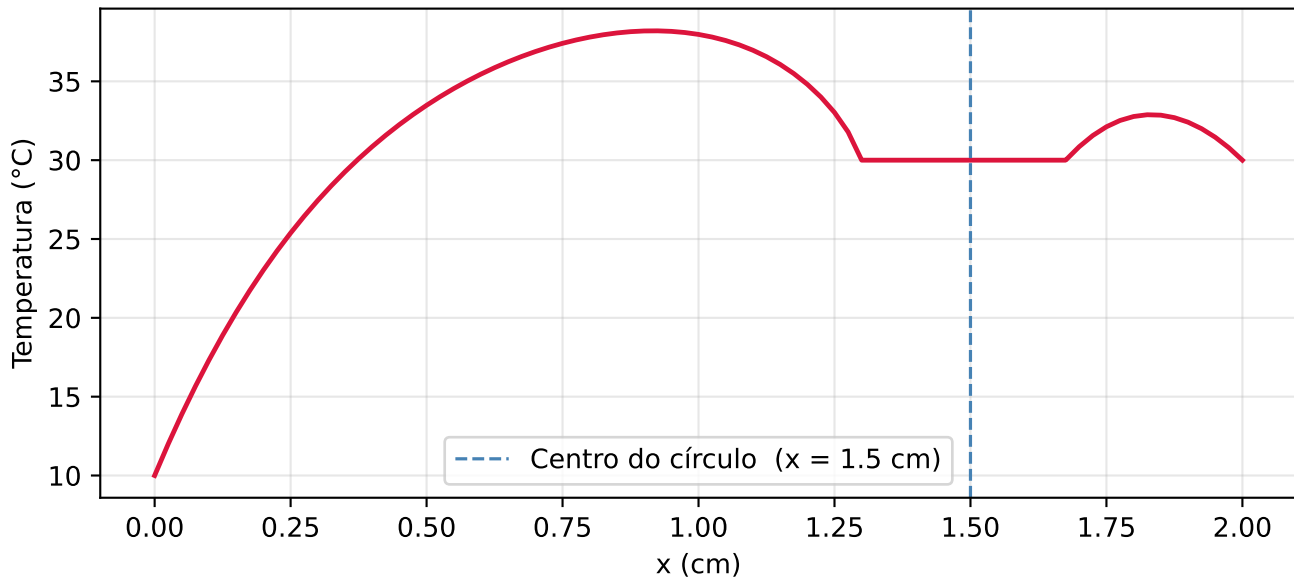
Perfil de temperatura - eixo central (81×41)
