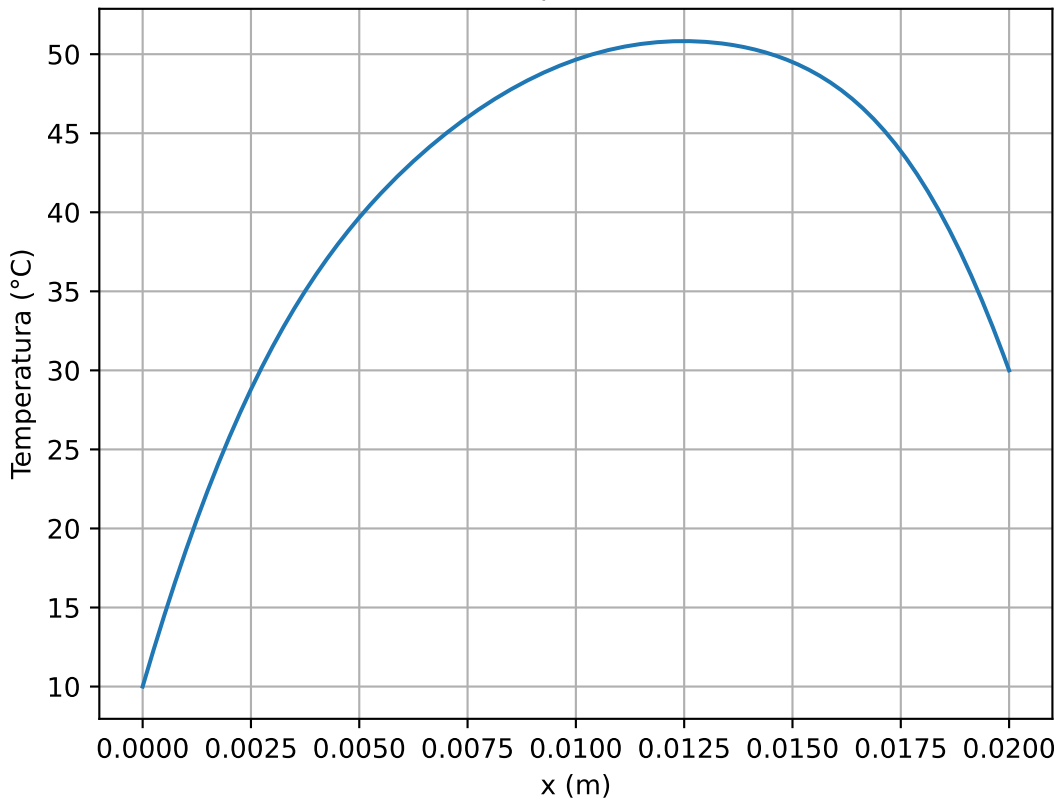
Eixo Central (161x81) | Temp. Máxima: 50.829 °C
