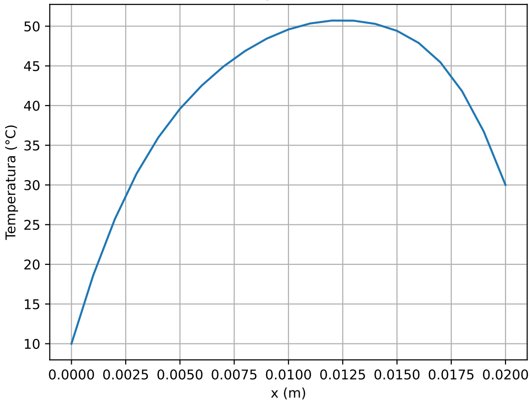
Eixo Central (21x11) | Temp. Máxima: 50.710 °C
