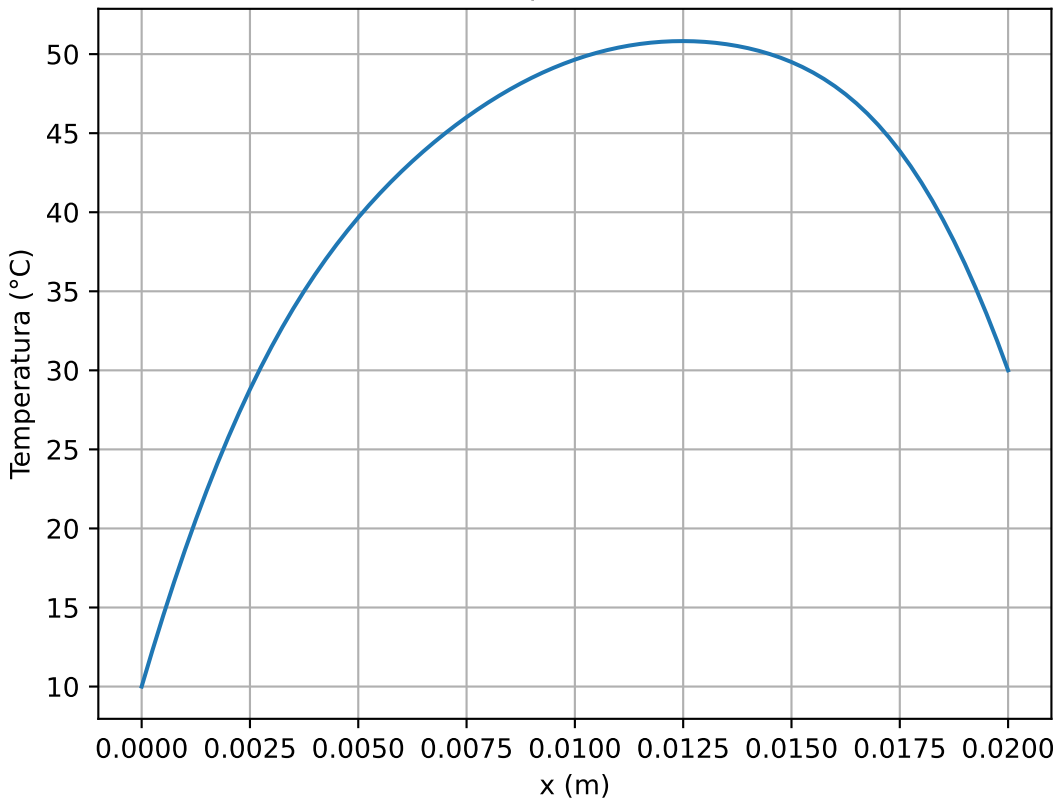
Eixo Central (81x41) | Temp. Máxima: 50.825 °C
