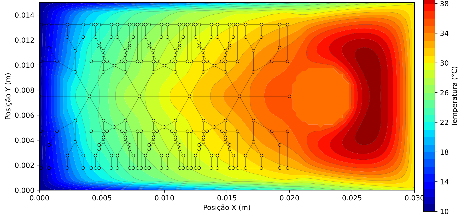
Campo Térmico 2D - Malha 121x61 | d_{max} = 0.001 m
