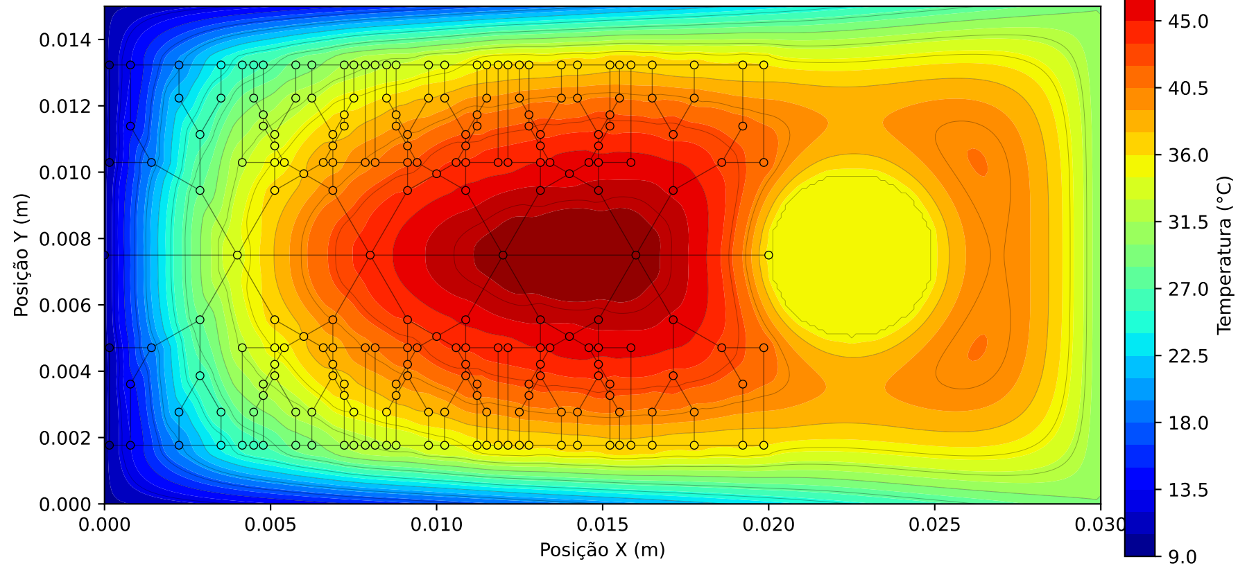
Campo Térmico 2D - Malha 241x121 | d_{max} = 0.00025 m
