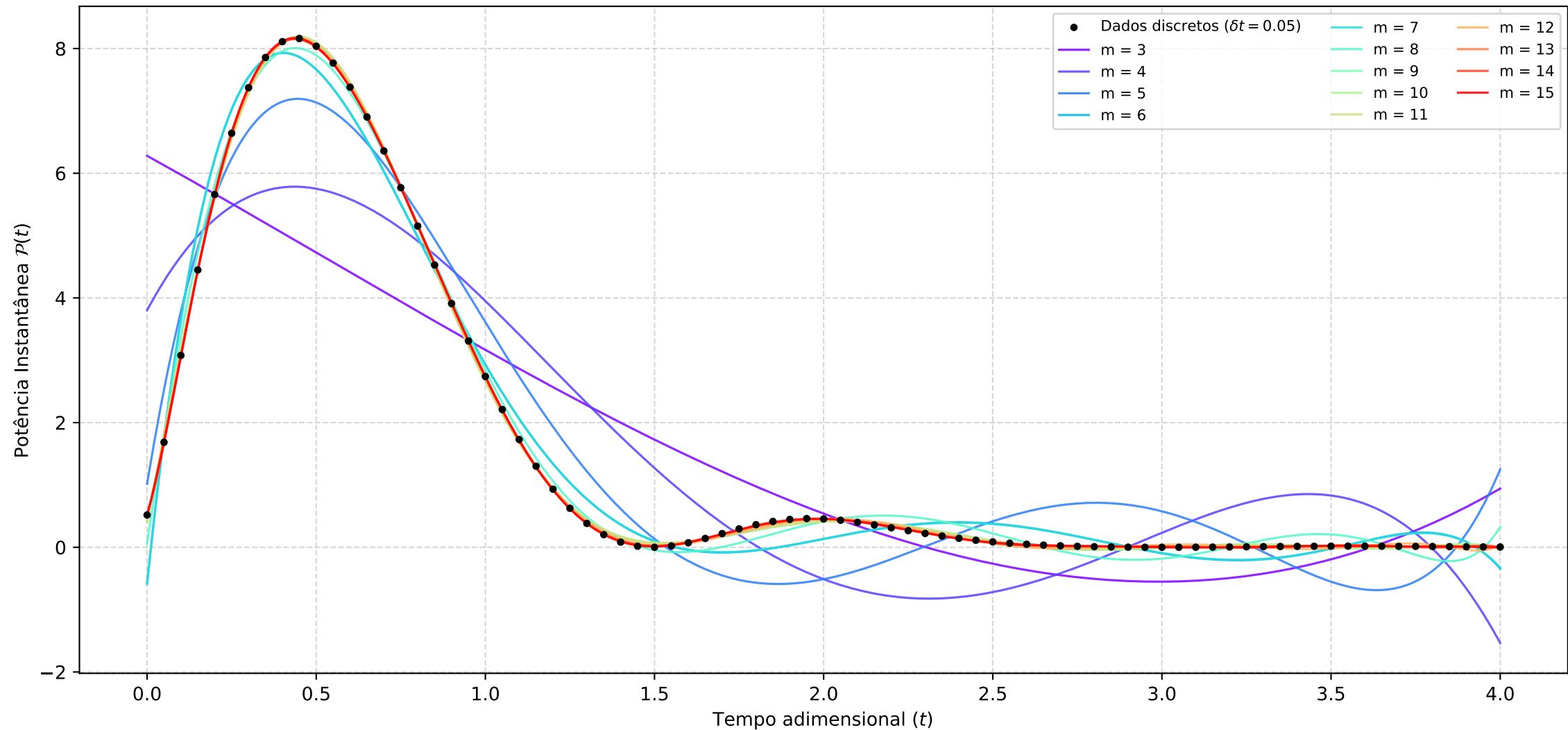
Regressão Polinomial Global — Graus m \in [3, 15]
