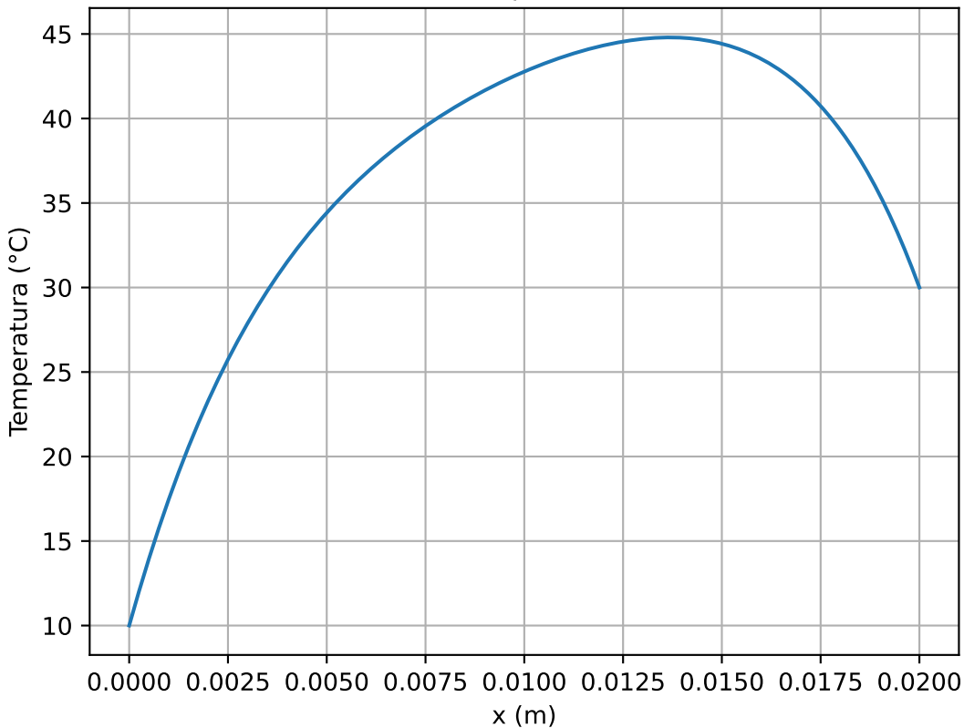
Eixo Central (321 X 161) | Temp. Máxima: 44.796 °C
