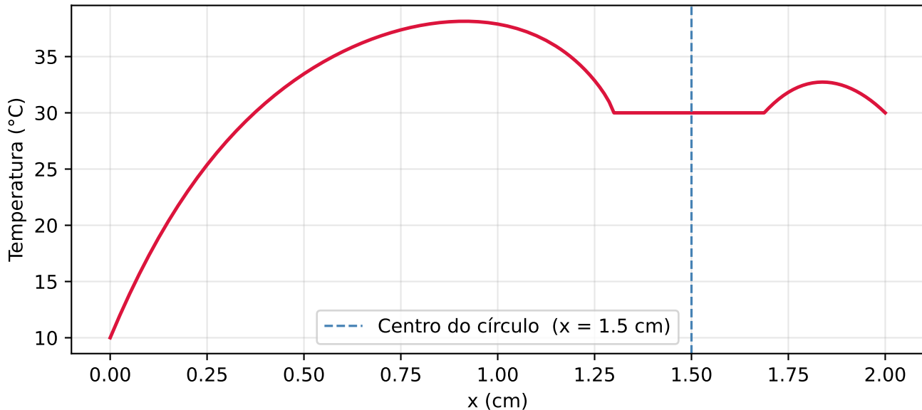
Perfil de temperatura - eixo central (161×81)
