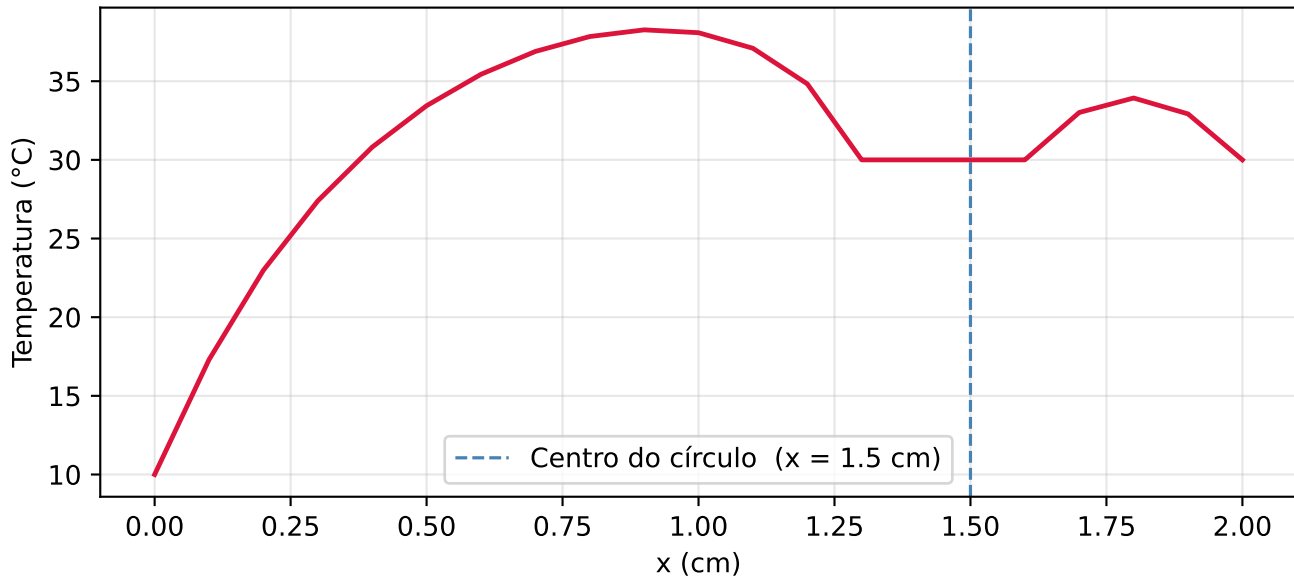
Perfil de temperatura - eixo central (21×11)
