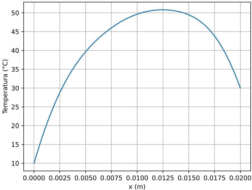
Eixo Central (41x21) | Temp. Máxima: 50.810 °C
