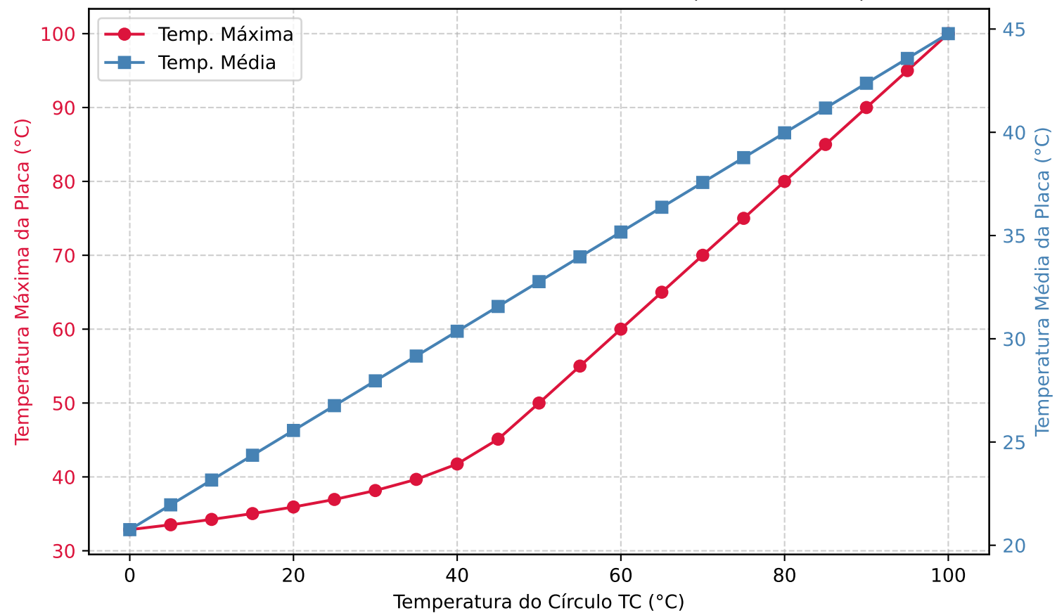
Estudo Paramétrico: Efeito de TC na Placa (Malha 101x51)
