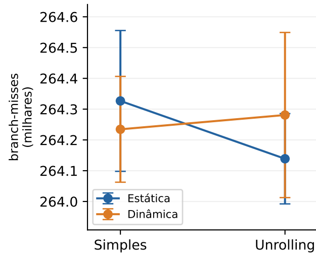
Interação: médias e IC95%
