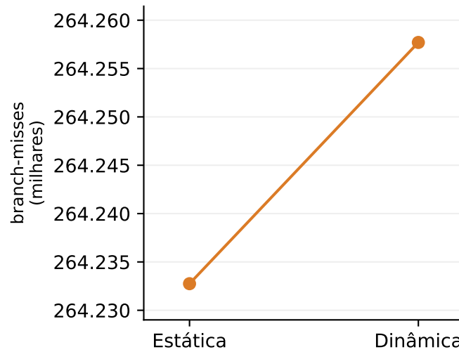
Efeito principal: alocação
