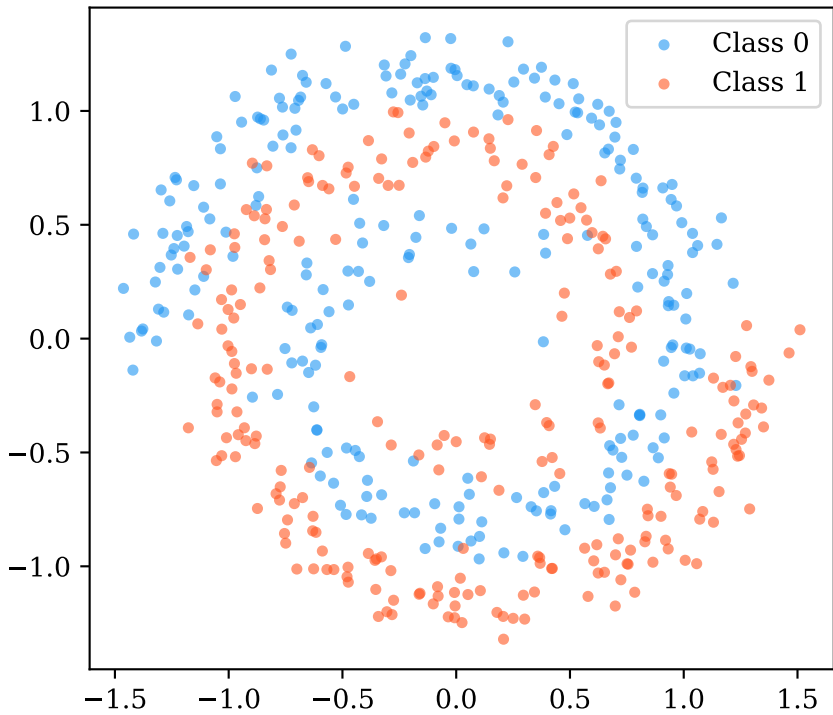
Dataset: spirals
