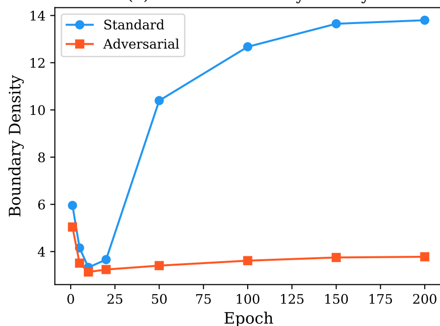
(d) Decision Boundary Density
