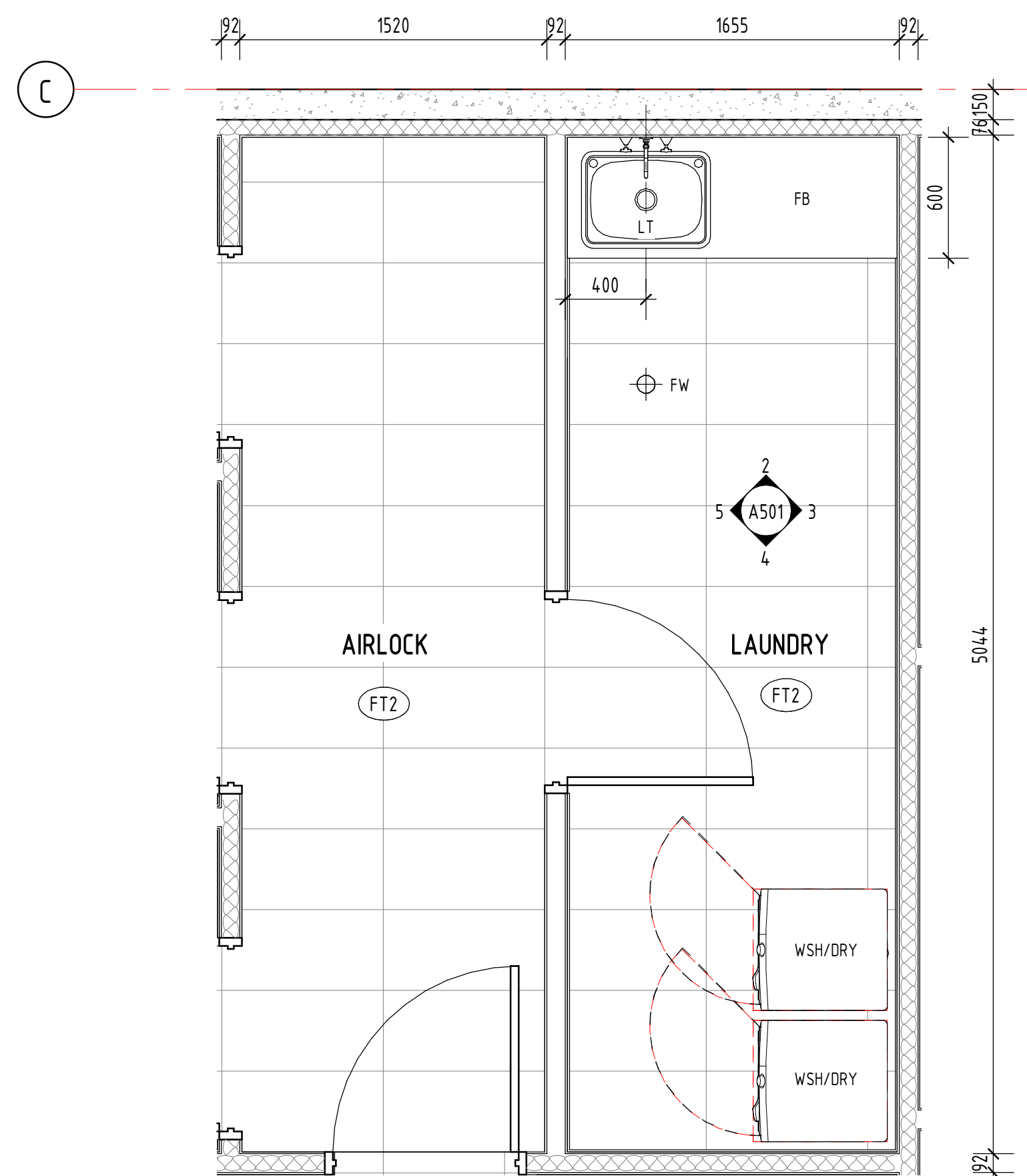
1 PROP. LAUNDRY PLAN 1 : 25
