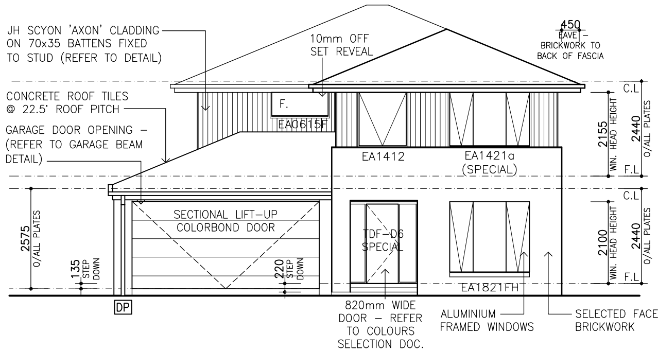
ELEVATION A
