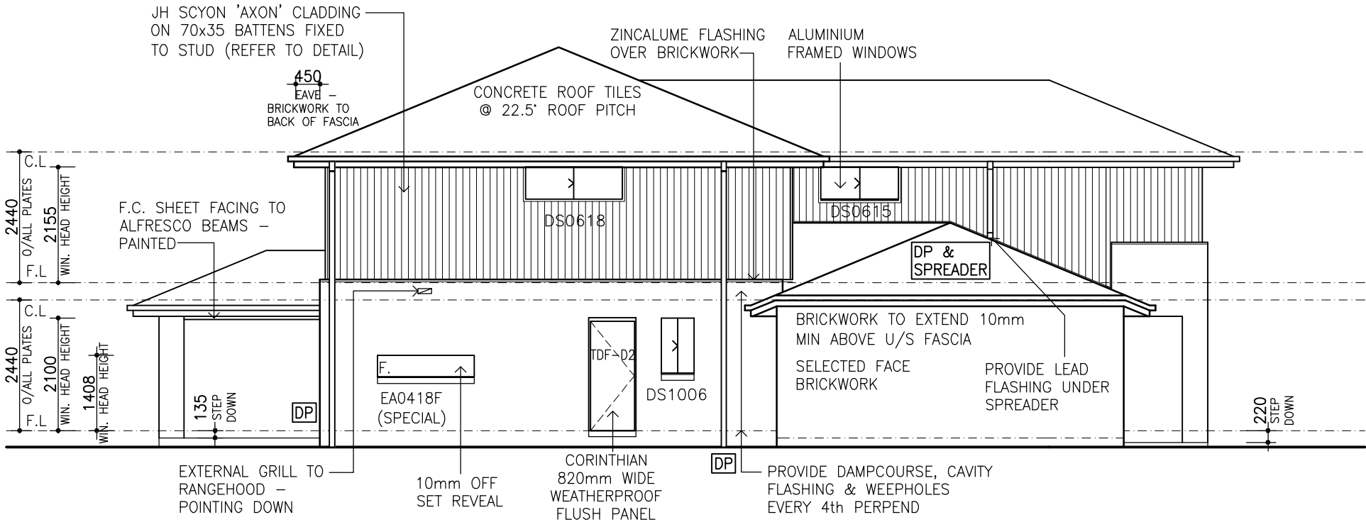
ELEVATION B
