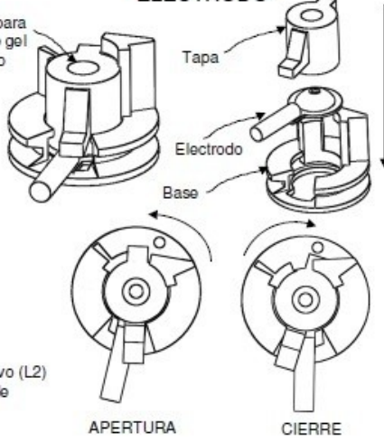
DETALLE DE FIJADOR DE ELECTRODO
