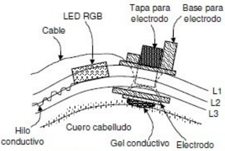
SISTEMA DE RETROALIMENTACIÓN HÁPTICO-VISUAL
