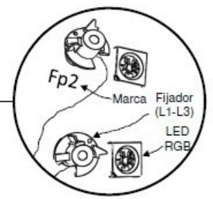
DETALLE DE FIJADOR DE ELECTRODO
