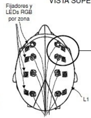
VISTA SUPERIOR DE GORRA
