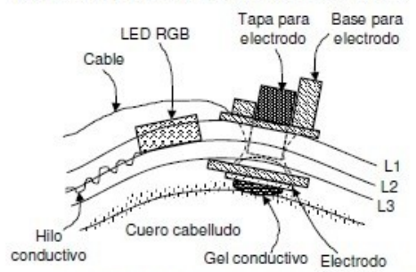
SISTEMA DE RETROALIMENTACIÓN HÁPTICO-VISUAL
