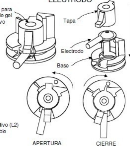
DETALLE DE FIJADOR DE ELECTRODO
