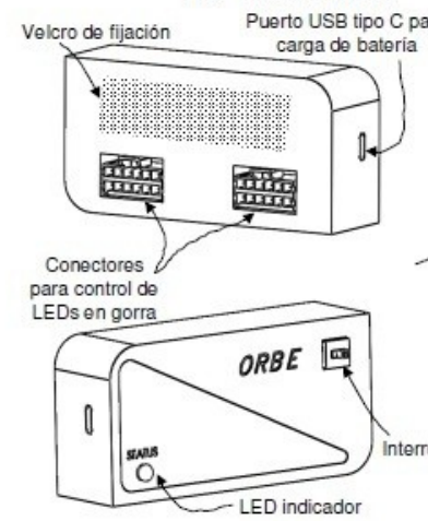
SISTEMA DE RETROALIMENTACIÓN HÁPTICO-VISUAL
