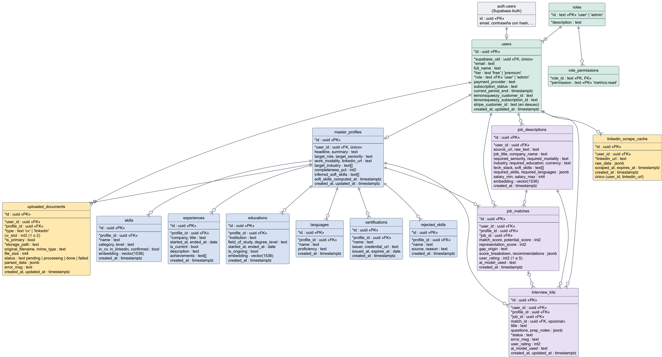
Modelo de datos de Jobby (esquema public de Supabase, 15 tablas)
