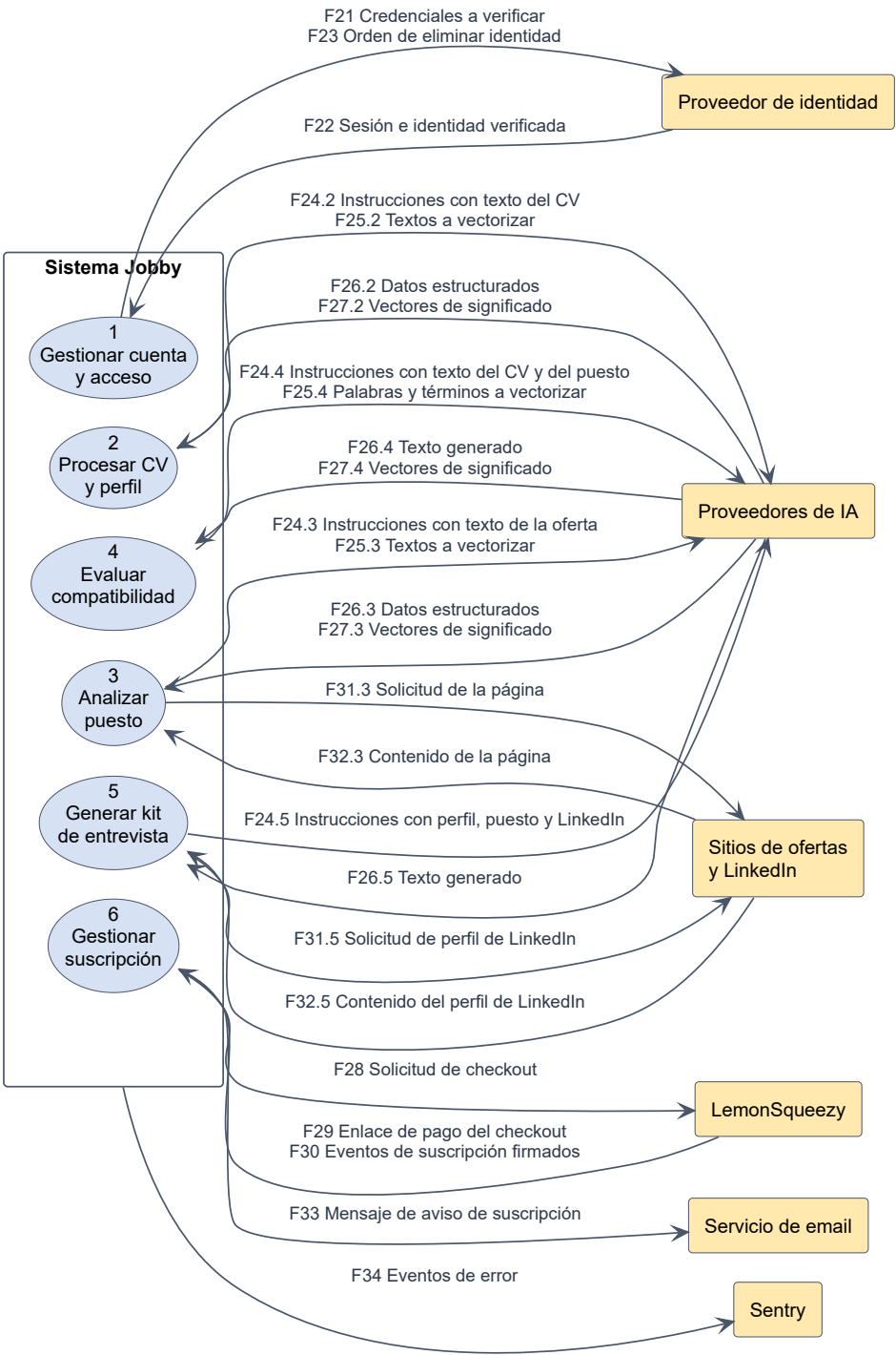
DFD nivel 1 — Vista 1B: procesos y sistemas externos
