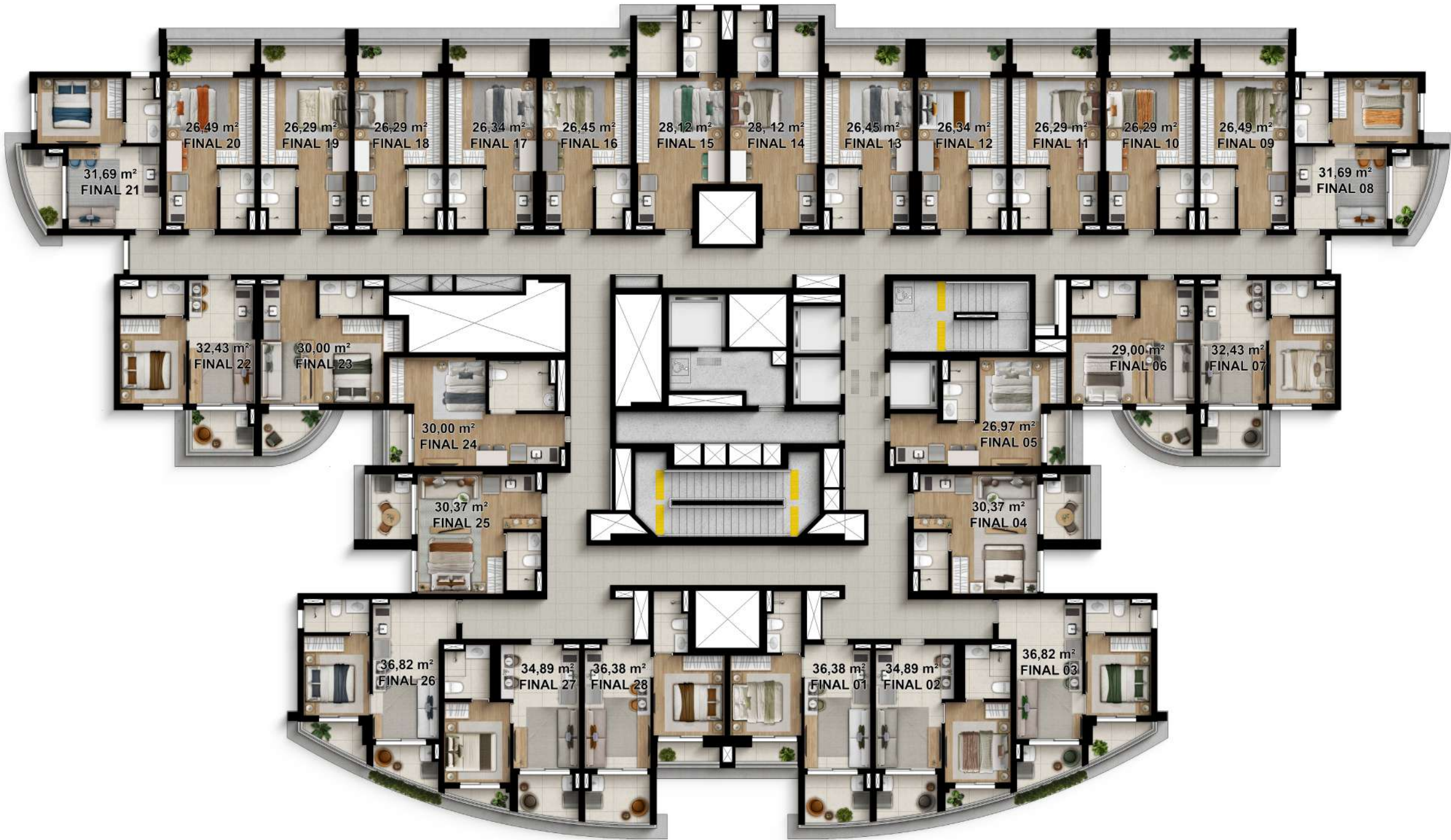
PLANTA 4° AO 10° PAVIMENTO
