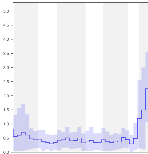
BDNN
