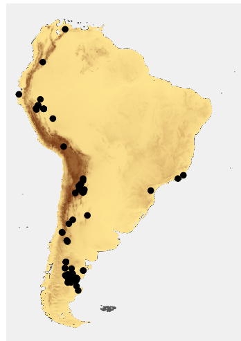
Pliocene
