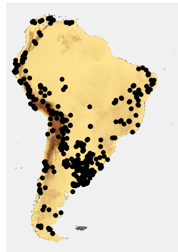
Pleistocene
