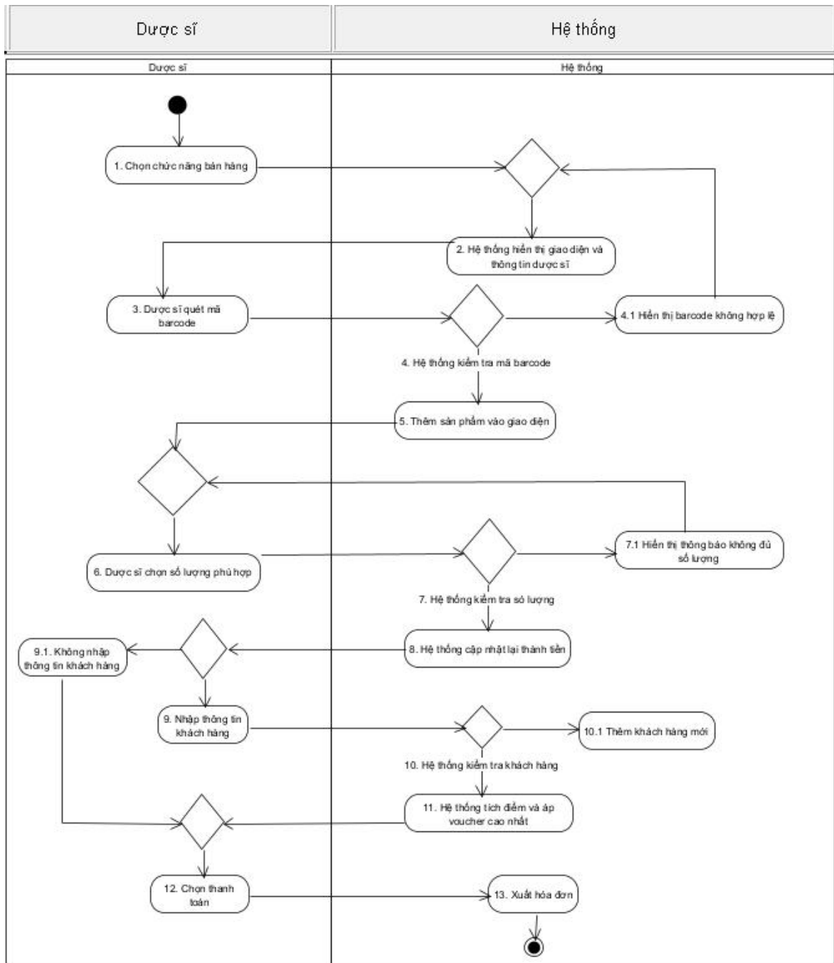
Hình 1. 4 Sơ đồ activity biểu diễn use case quản lý bán hàng
