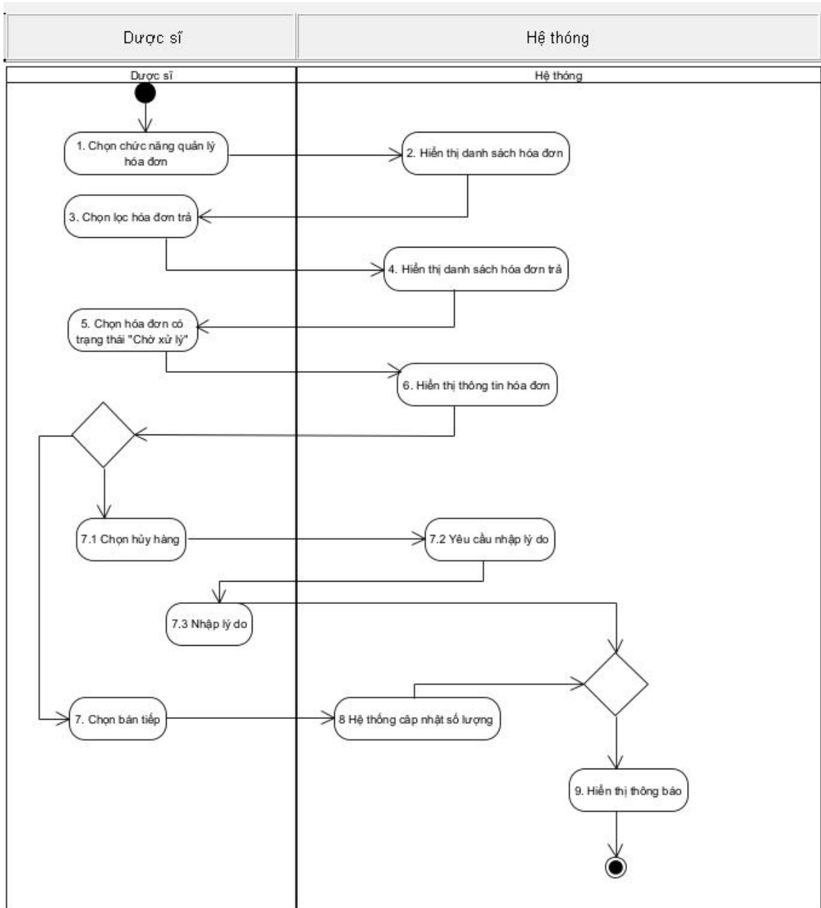
Hình 1. 8 Sơ đồ activity biểu diễn chức năng quản lý hàng đổi trả
