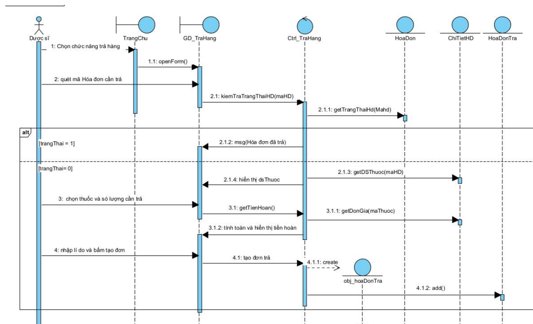
Hình 1. 7 Sơ đồ sequence biểu diễn chức năng trả hàng
