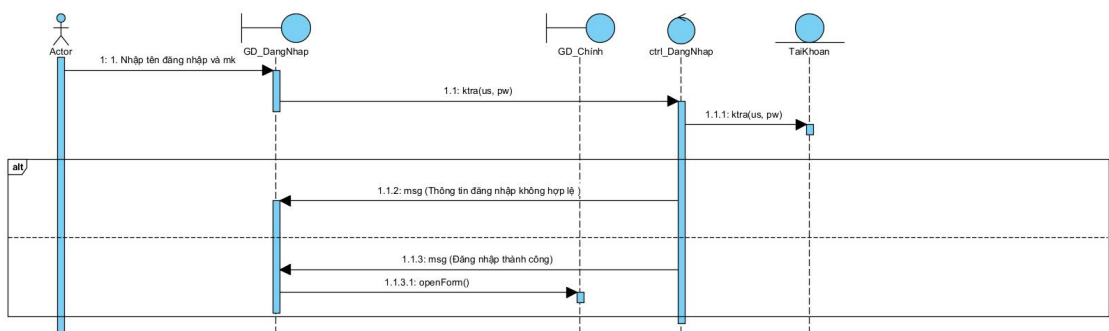
Hình 1. 3 Sơ đồ Sequence biểu diễn chức năng đăng nhập
