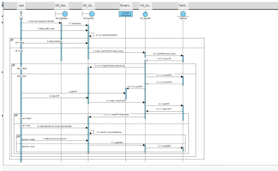
Hình 1. 13 Sơ đồ sequence biểu diễn chức năng quên mật khẩu
