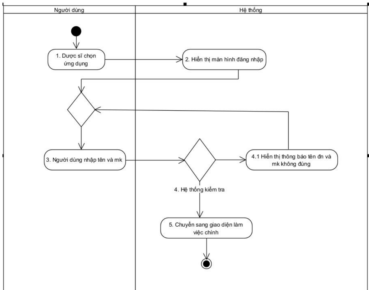
Hình 1. 2 Sơ đồ activity đăng nhập
