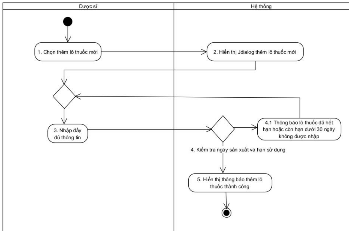
Hình 1. 10 Sơ đồ activity biểu diễn chức năng quản lý lô thuốc
