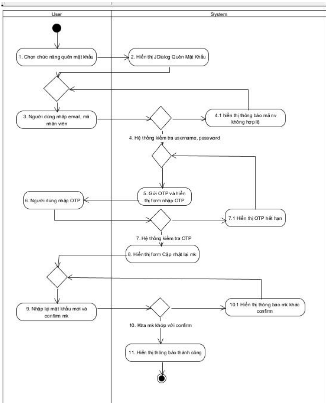
Hình 1. 12 Sơ đồ activity biểu diễn chức năng quên mật khẩu
