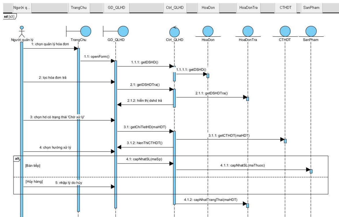
Hình 1. 9 Sơ đồ sequence biểu diễn chức năng quản lý hàng đổi trả
