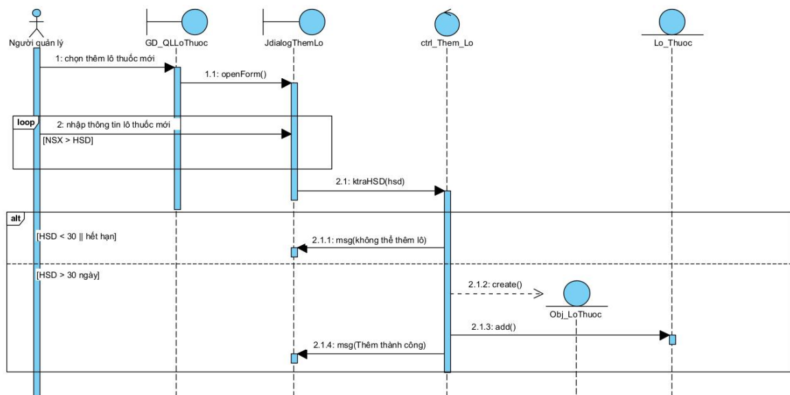
Hình 1. 11 Sơ đồ sequence biểu diễn chức năng quản lý lô hàng
