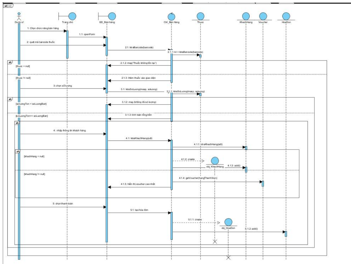
Hình 1. 5 Sơ đồ sequence biểu diễn chức năng bán hàng
