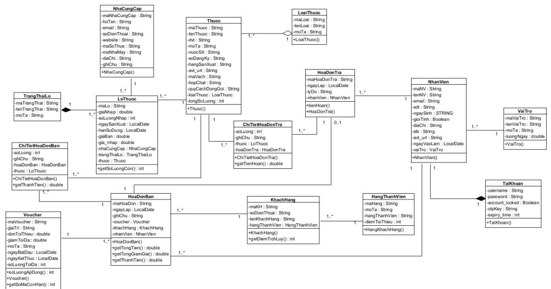
Hình 1. 14 Sơ đồ lớp của hệ thống quản lý hiệu thuốc tây
