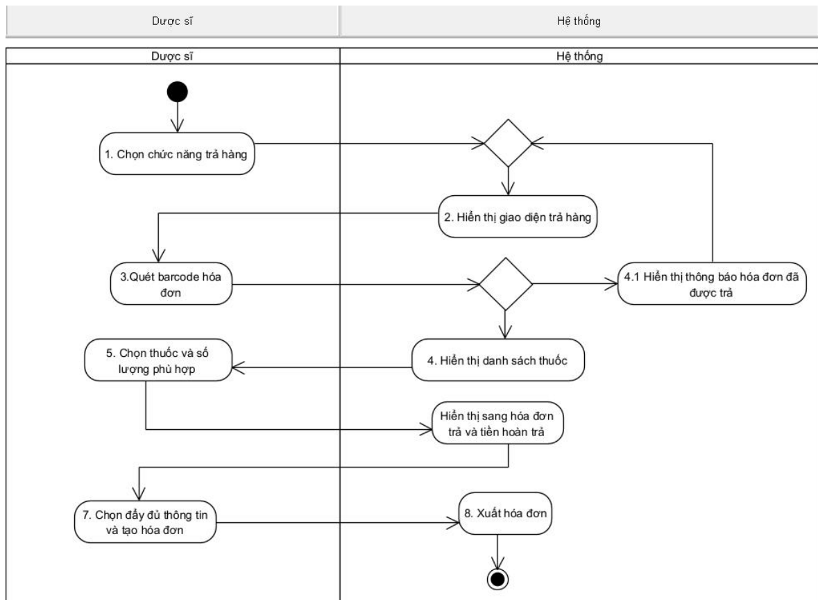
Hình 1. 6 sơ đồ activity biểu diễn chức năng trả hàng
