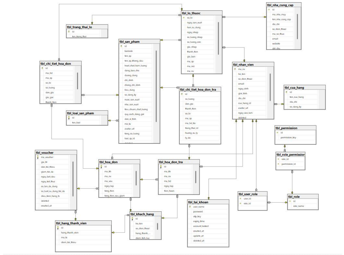
Hình 1. 16. Mô hình cơ sở dữ liệu quan hệ của nhà thuốc Alami
