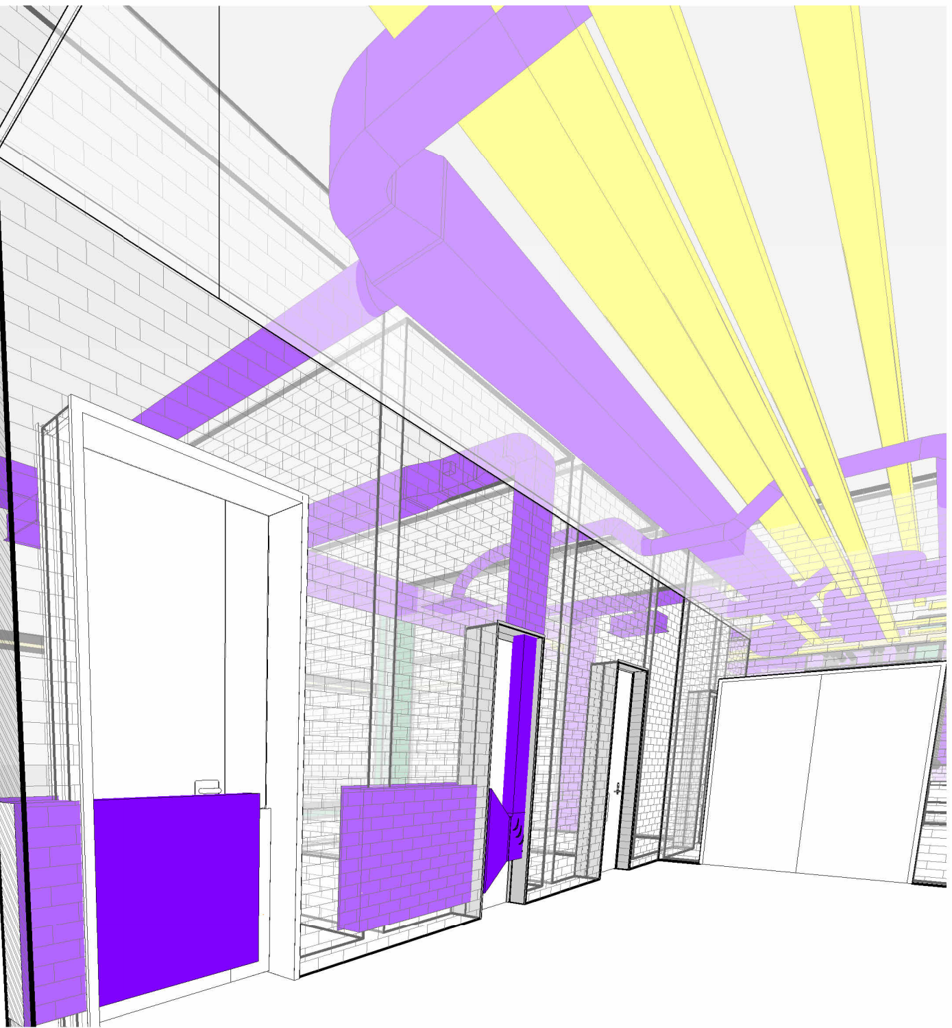
Passage HVAC Clash
