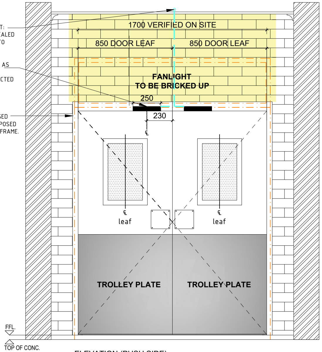
ELEVATION (PUSH SIDE)
