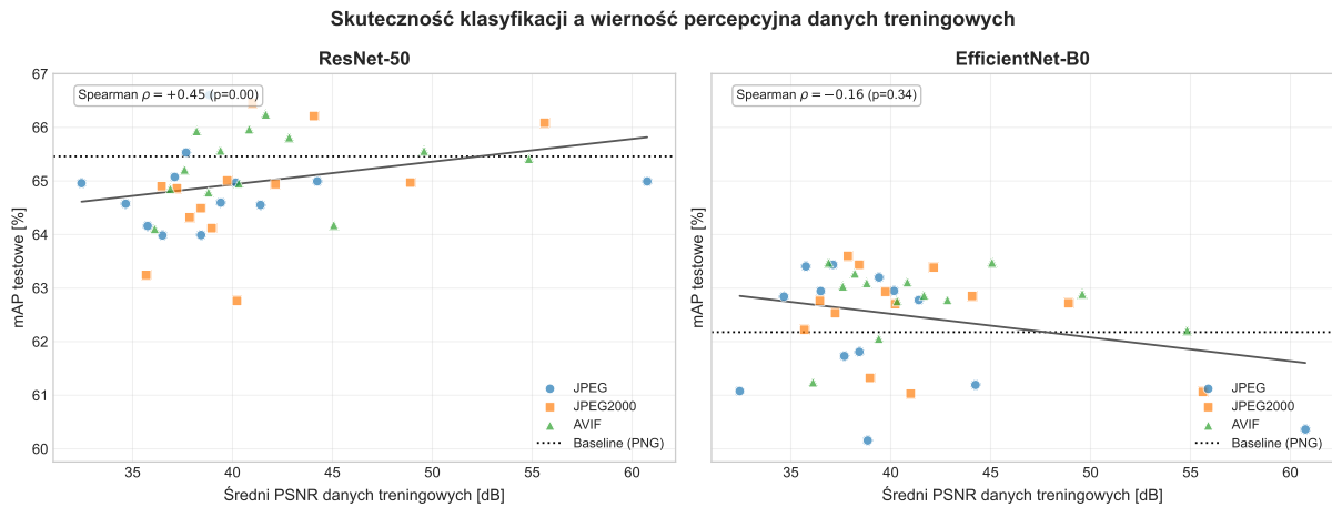
Rysunek 4: Skuteczność klasyfikacji (mAP testowe) w funkcji średniej wierności percepcyjnej danych treningowych (PSNR). Brak spójnego dodatniego trendu między architektu-rami wskazuje, że PSNR/SSIM nie są dobrym predyktorem skuteczności w tym zadaniu.
