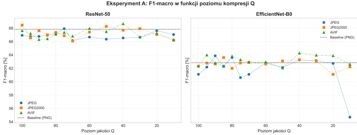
Rysunek 3: Eksperyment A: F1-macro w funkcji poziomu kompresji Q dla obu architektur; pozioma linia przerywana oznacza model bazowy (PNG).
