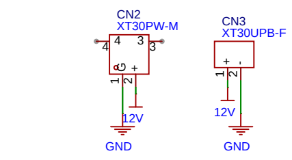
XT30供电
