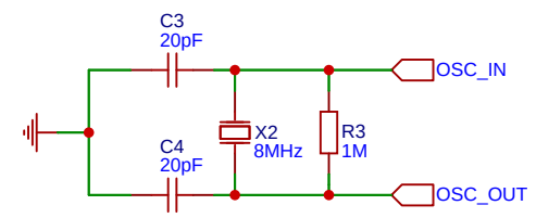
外部晶振
