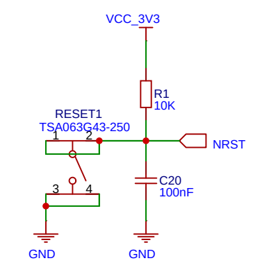
复位按键
