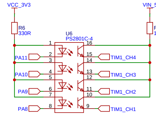
光耦隔离
