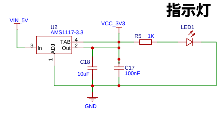
3.3V稳压输出
