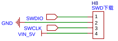
SWD下载口
