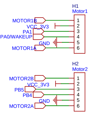
电机接口
