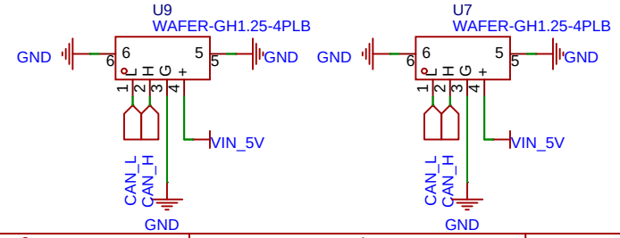
CAN接口
