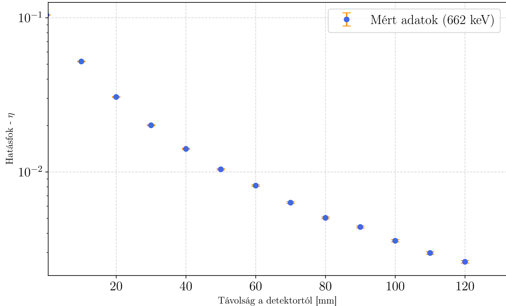
Detektor csúcshatásfoka a forrás távolságának függvényében
