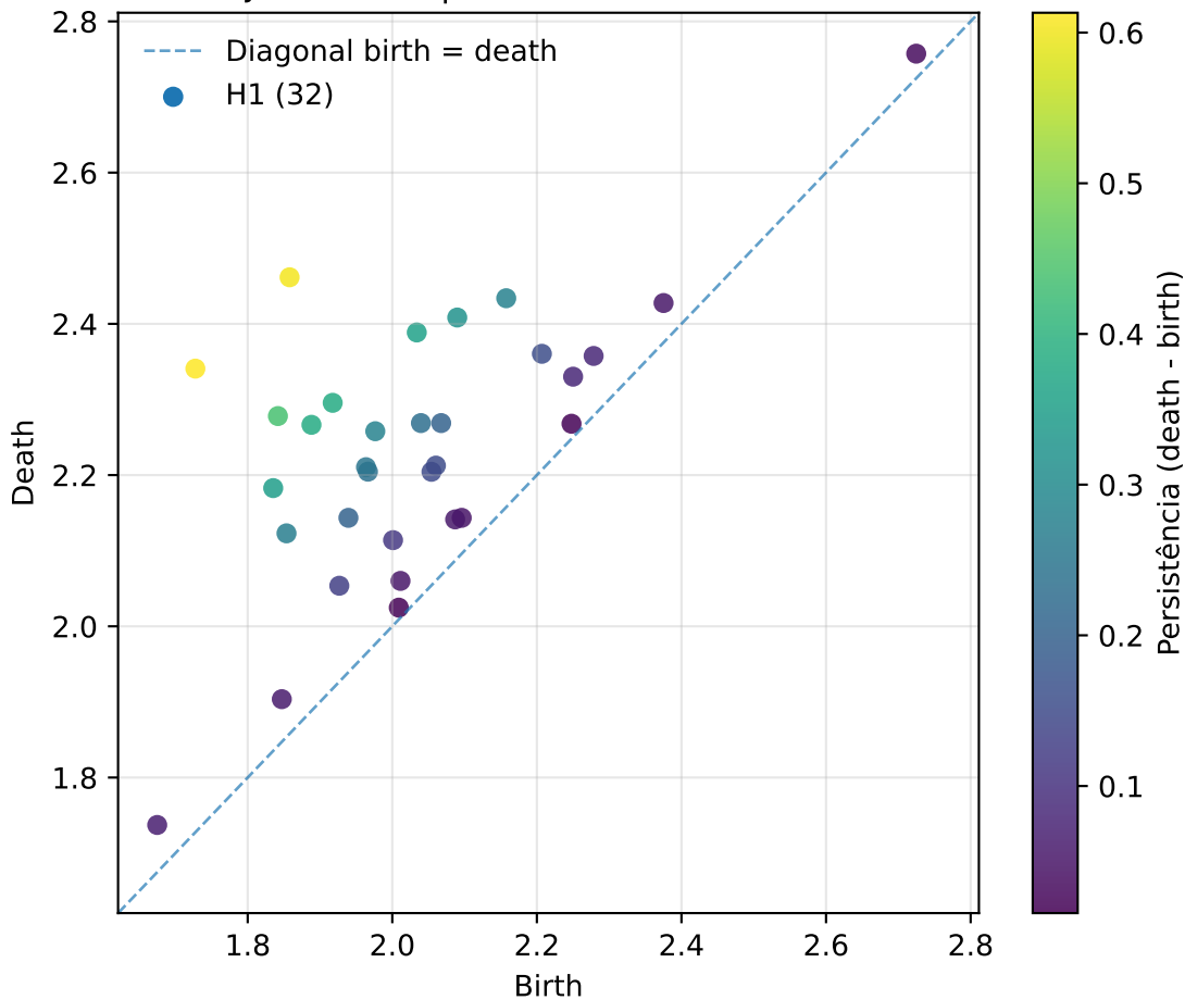
Diagrama de persistência — ABEV3.SA janela 188 | referência 2014-01-17
