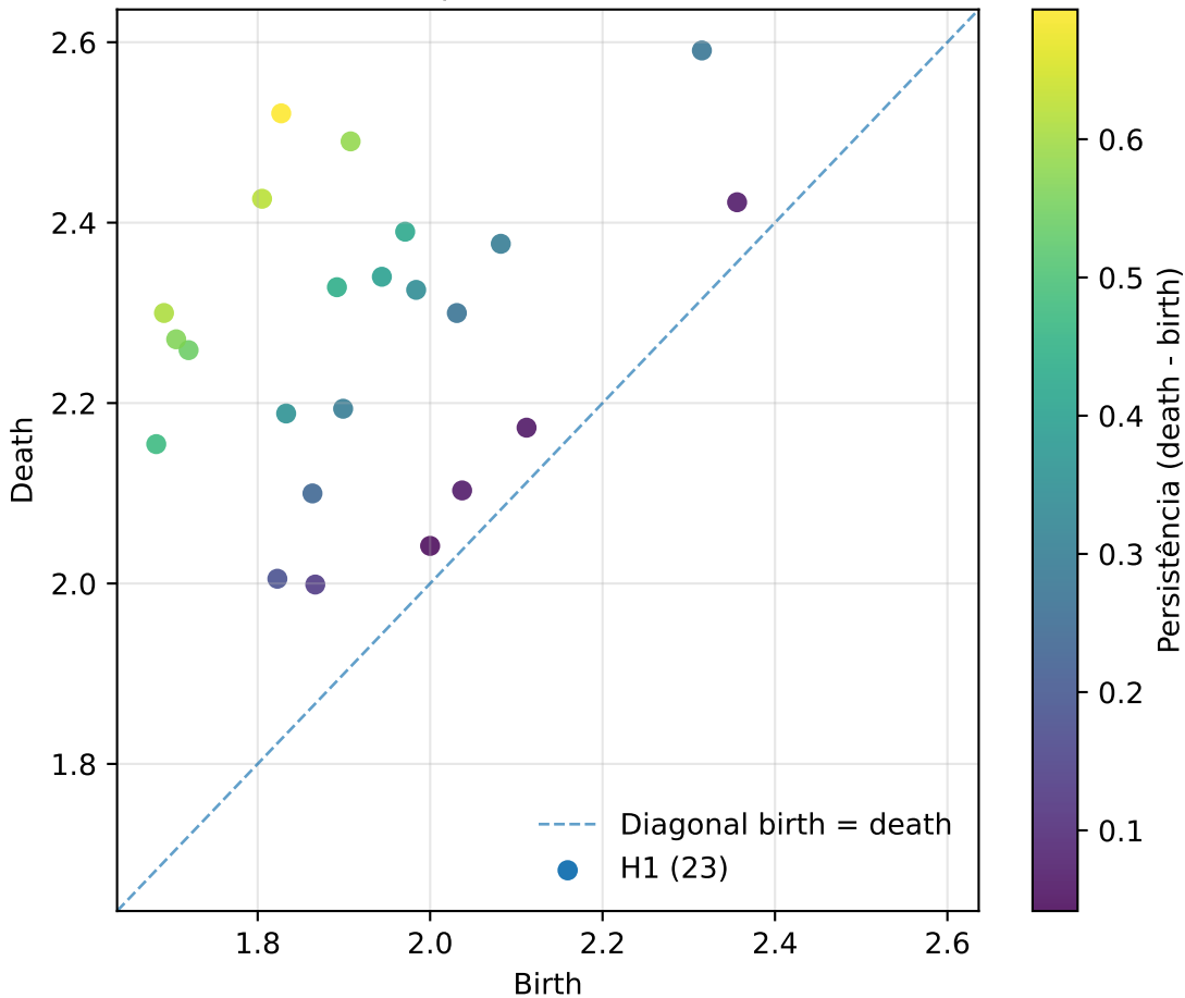
Diagrama de persistência — ITUB4.SA janela 778 | referência 2025-11-25
