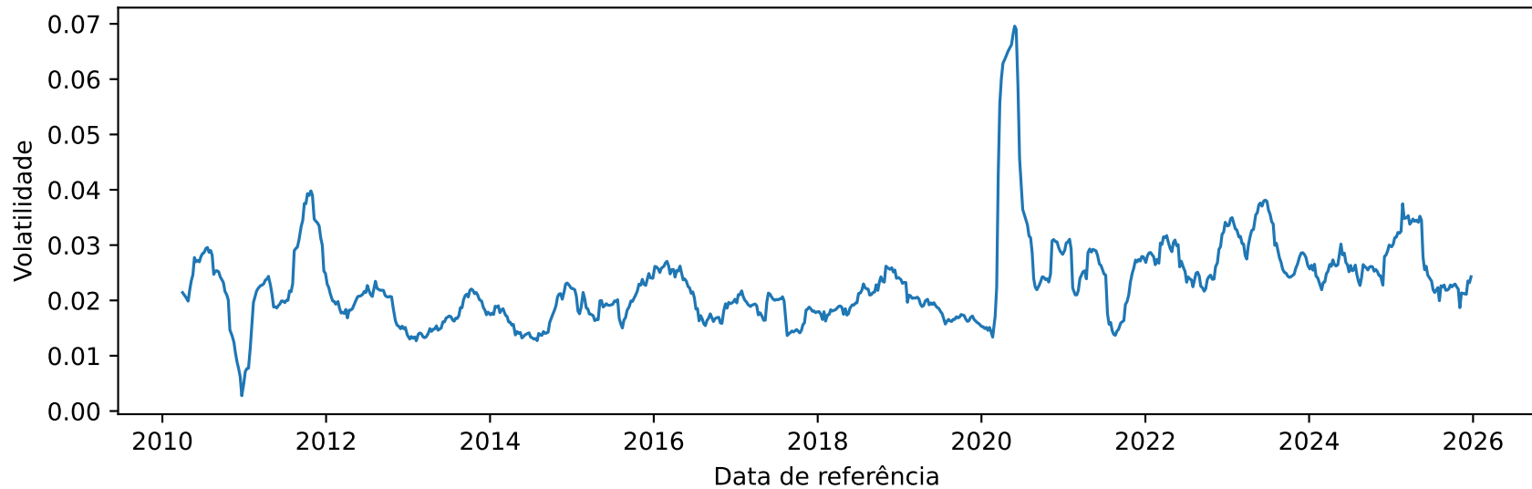
Volatilidade por janela — LREN3.SA
